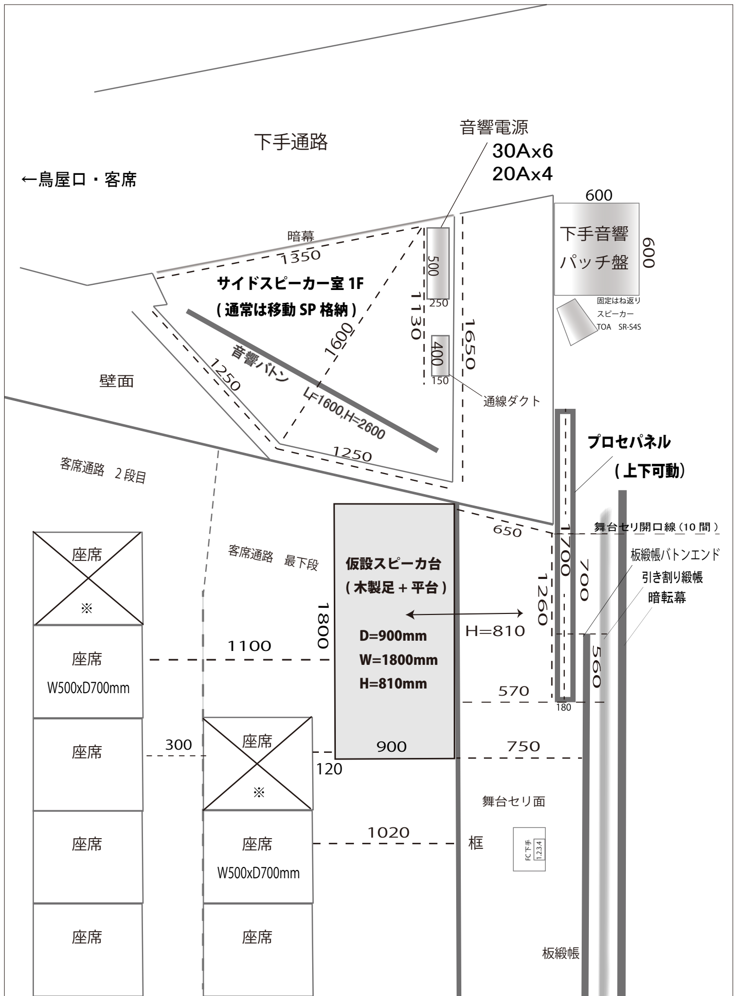
由利本荘市文化交流館カダーレ・ホール スピーカー設置スペース寸法図
